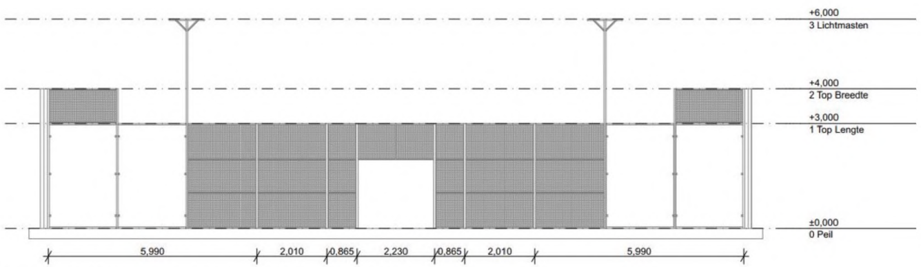
Figuur 5-1: Vooraanzicht padelkooi
