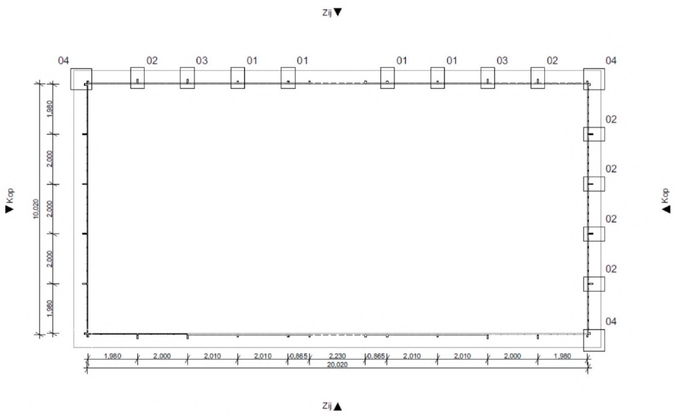
Figuur 5-3: plattegrond standers padelkooi
