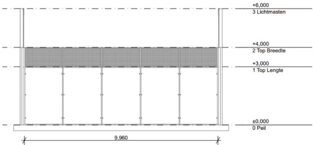
Figuur 5-2: Zijaanzicht padelkooi
